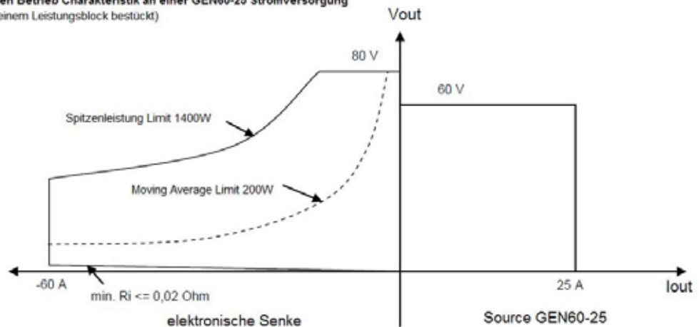
Senken Betrieb Charakteristik an einer GEN60-25 Stromversorgung (mit einem Leistungsblock bestückt)
